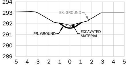
STA. 1+500
