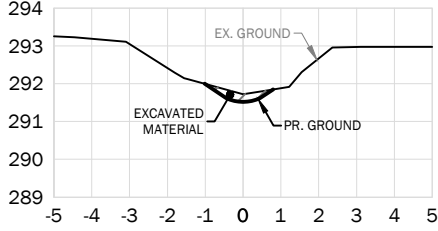
STA. 1+450
