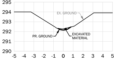
STA. 1+800
