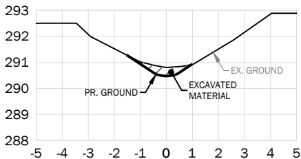
STA. 0+300
