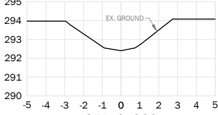
STA. 1+900
