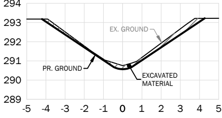
STA. 0+450
