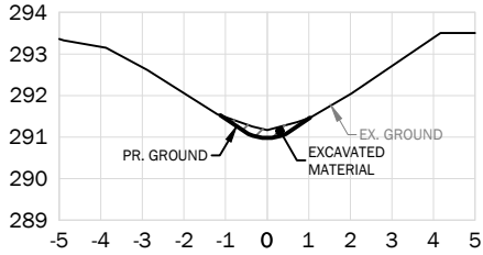
STA. 1+050
