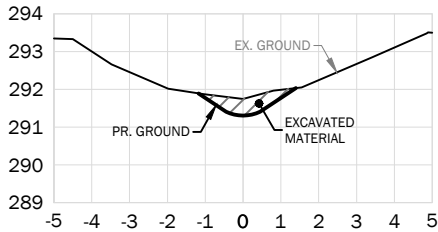
STA. 1+300
