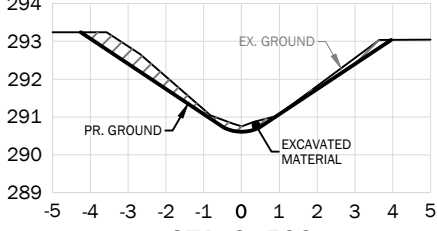
STA. 0+500
