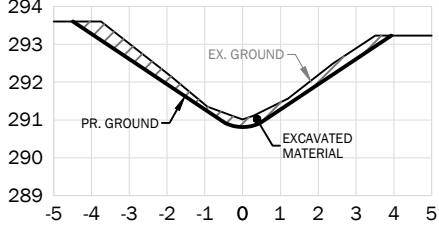
STA. 0+800
