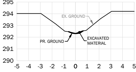
STA. 1+850
