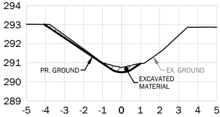
STA. 0+350
