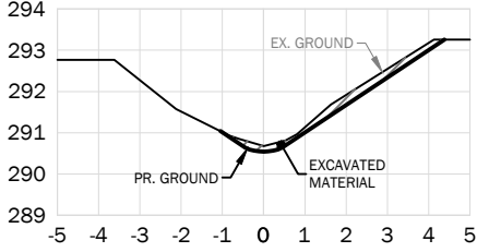
STA. 0+400
