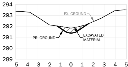
STA. 1+350
