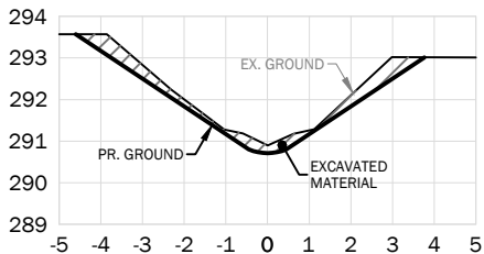
STA. 0+650
