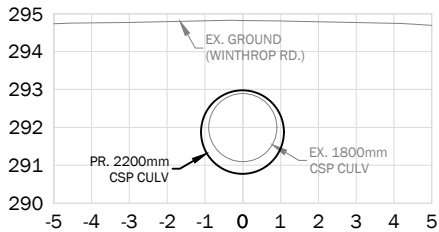
STA. 0+950
