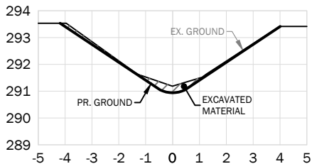
STA. 1+000
