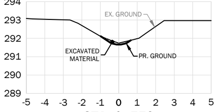
STA. 1+550
