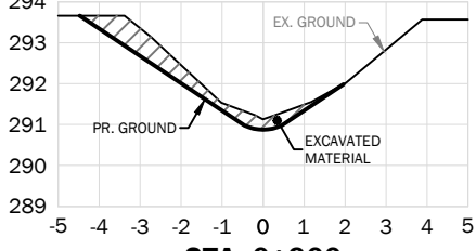
STA. 0+900
