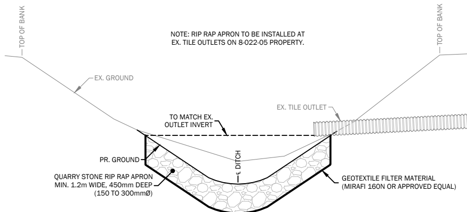
TYPICAL RIP RAP APRON DETAIL N.T.S.
