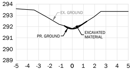
STA. 1+650
