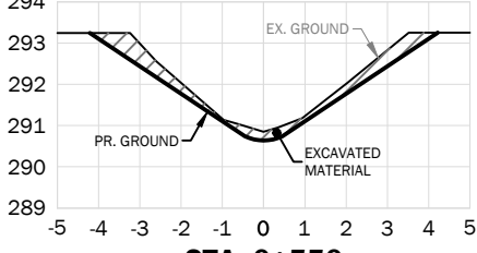
STA. 0+550
