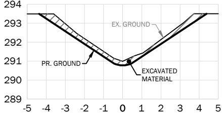
STA. 0+750
