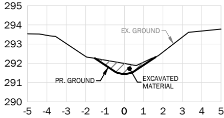
STA. 1+400
