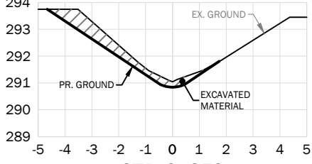
STA. 0+850
