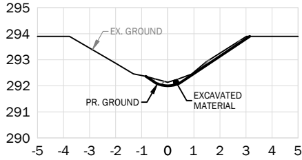
STA. 1+750
