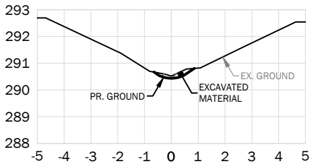
STA. 0+250
