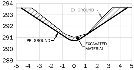
STA. 0+700
