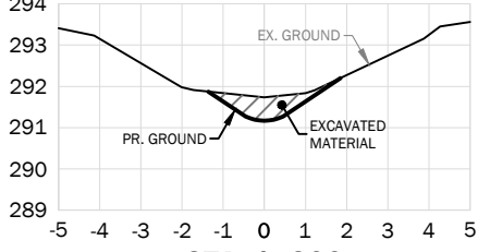
STA. 1+200
