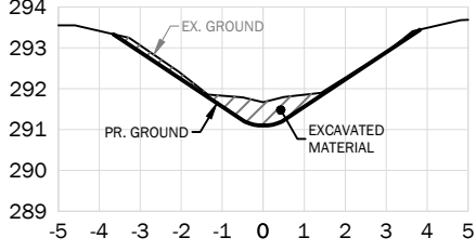
STA. 1+150
