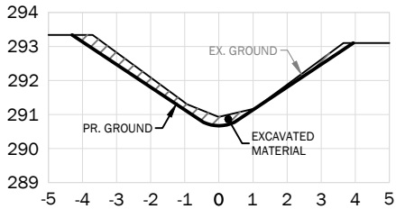
STA. 0+600
