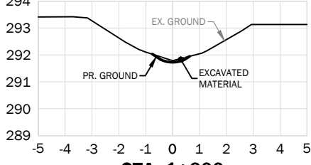
STA. 1+600
