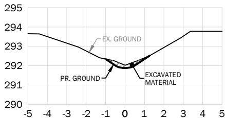
STA. 1+700
