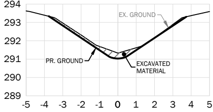
STA. 1+100
